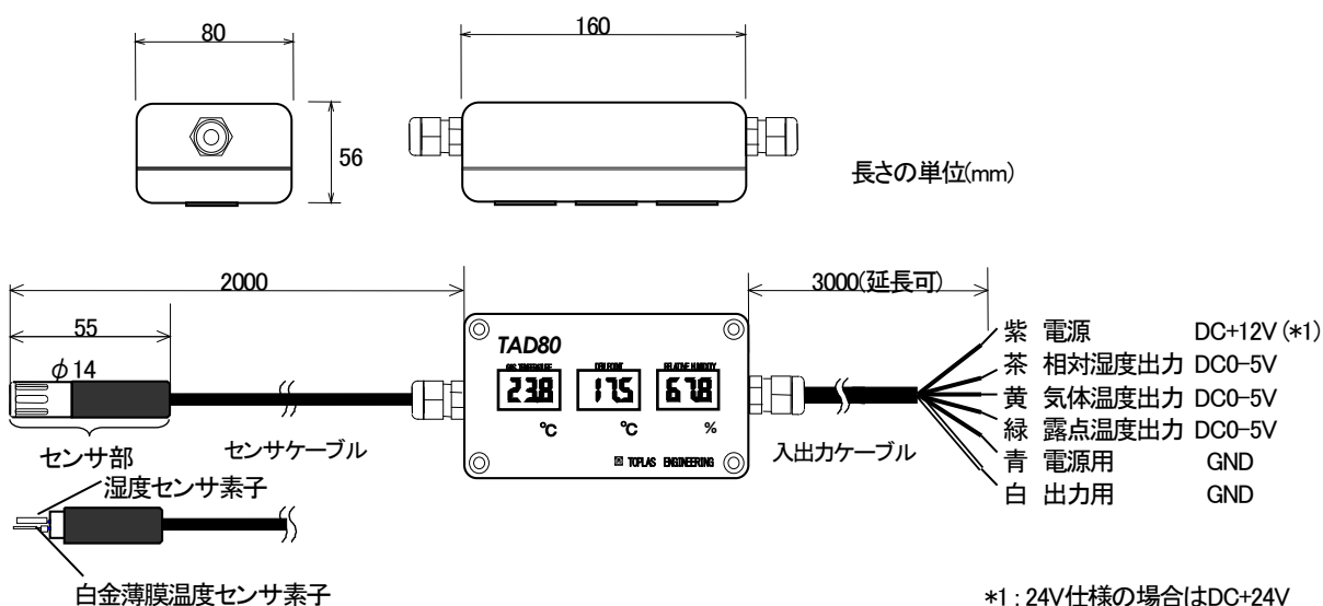
図1 TAD801L および TAD802L の外形および配線
