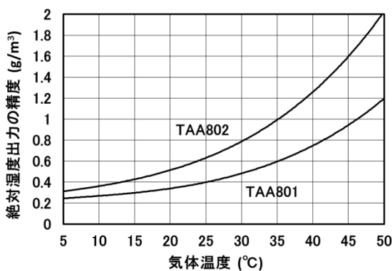
5~50°Cの場合 50~95°Cの場合 図2 絶対湿度の計測精度 (広範囲型 電圧出力に於いて)
