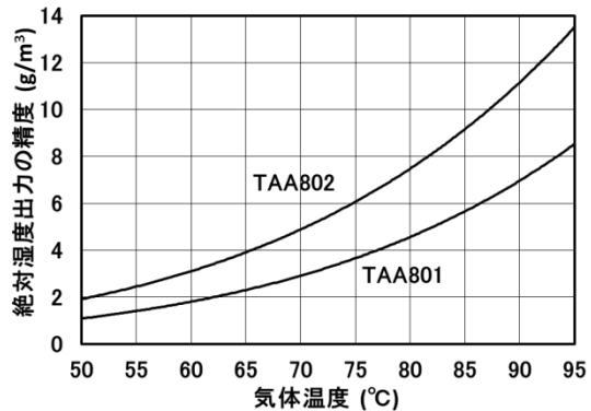
5~50°Cの場合 50~95°Cの場合 図2 絶対湿度の計測精度 (高精度型 電圧出力に於いて)
